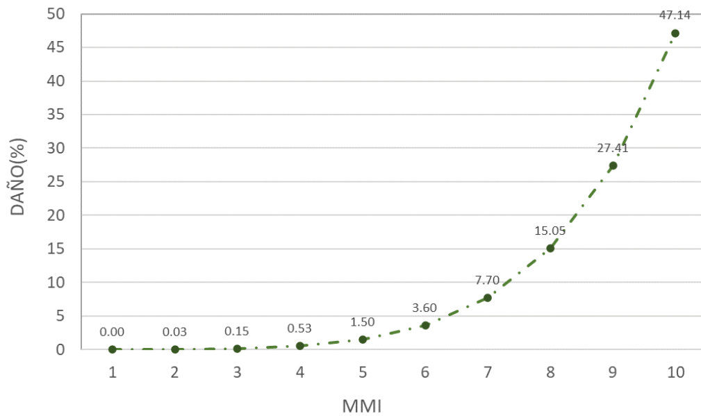
Gráfica 6.1. Curva de danos para edificios da Administración estatal, autonómica, comarcal e local (F10)
