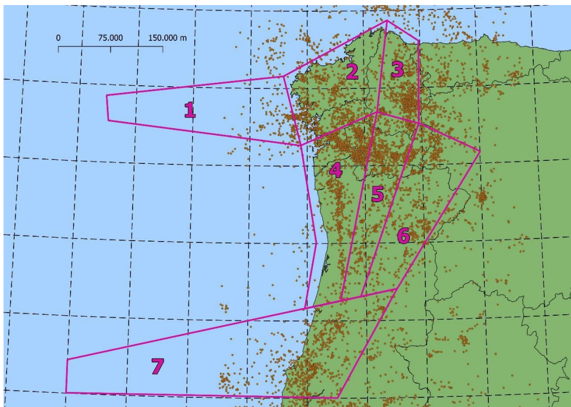
Figura 2.5. Zonas sísmoxénicas consideradas na NCSE-02
