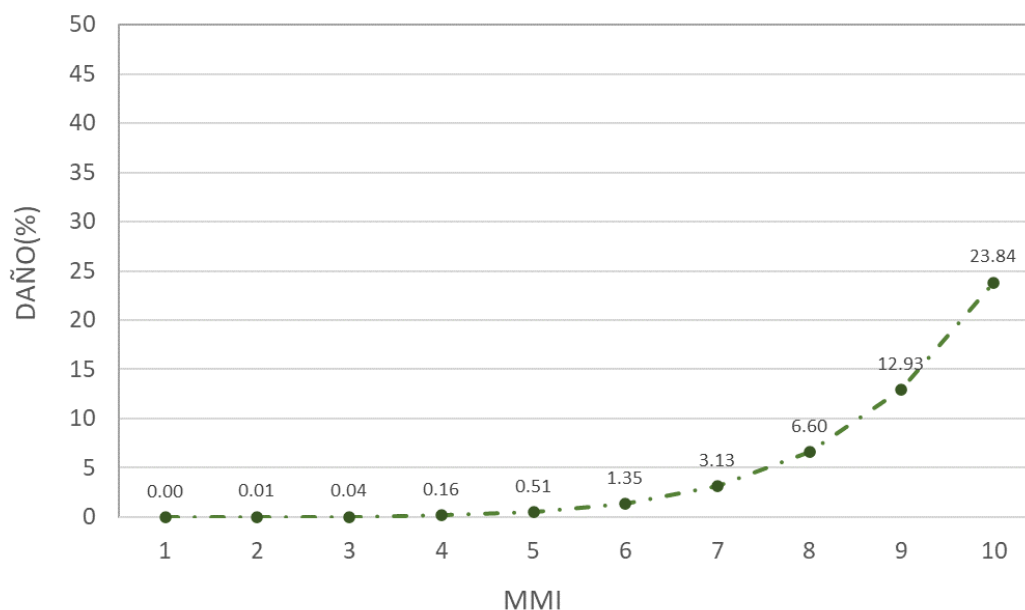
Gráfica 6.17. Curva de danos para os parques industriais (FC12+FC68+FC49)
