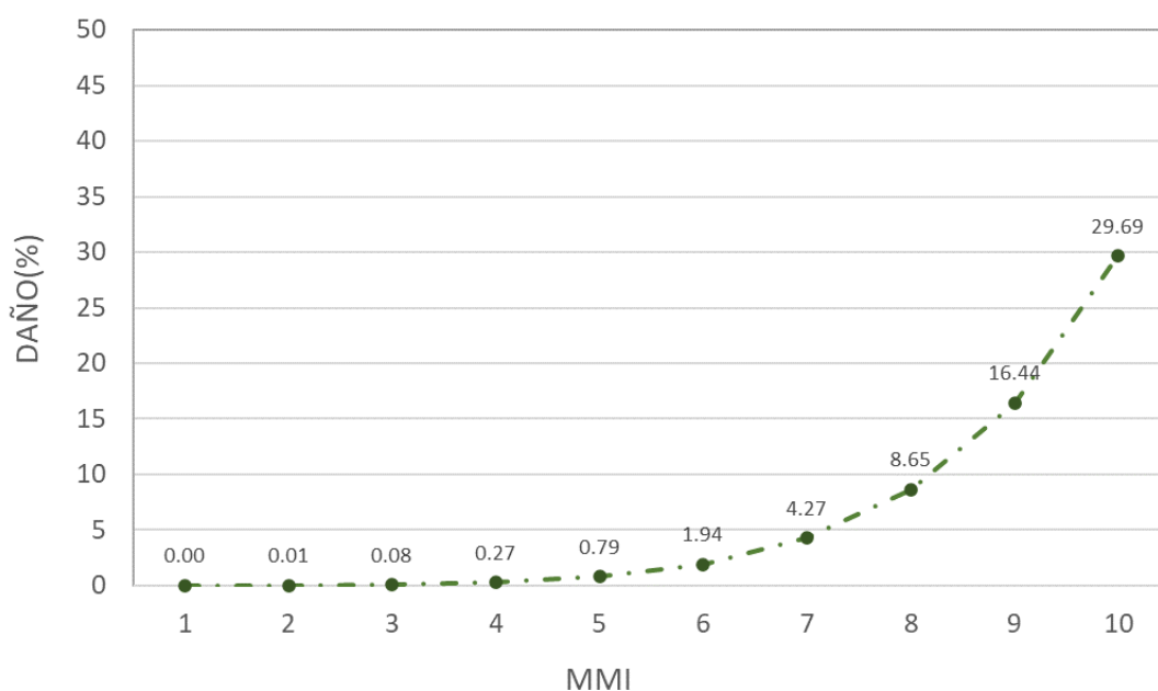
Gráfica 6.10. Curva de danos para as estacións de autobuses (FC10+FC90+FC49)
