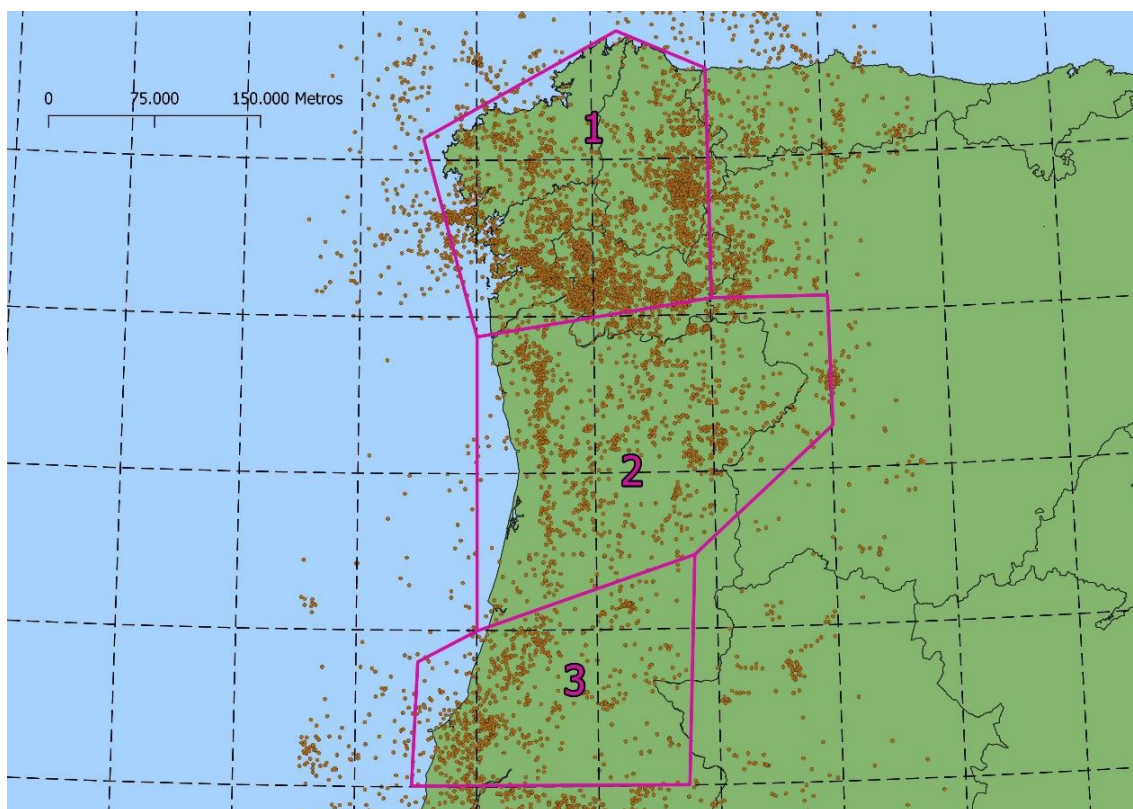
Figura 2.4. Zonas sismoxénicas consideradas na NCSE-94
